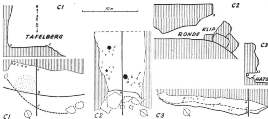
Fig. 6. Platte grond en doorsnede van de vindplaatsen bij de Tafelberg van Santa Barbara (C 1), op Ronde Klip (C 2) en bij Hato (C 3), Curaçao . — De kalksteenrots is gearceerd; de verweerde druipsteen zuilen zijn massief zwart. De rand van het overhangende deel is met een gesloten lijn aangeduid; belangrijke reliëfverschillen van de bodem met een gebro- ken lijn. De hoofdletters hebben betrekking op de plaats waar de door- snede is gemaakt; de kleine cursieve letters op de ligging van de afge- beelde tekeningen; de v-tekentjes op die van onduidelijke resten. Fig. 6. Ground plan and cross section of the Tafelberg (C 1), Ronde Klip (C 2) and Hato (C 3) localities, Curaçao . — Coral rock striped; pillars of weathered dripstone indicated by black dots; figures by a, b, c, etc.; vague remnants of red figures by v-v.
